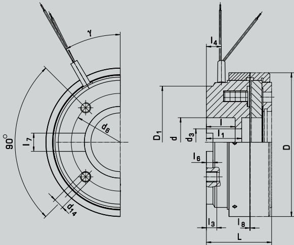
Magnetteilbauform 3, mit freien Anschlusskabeln
