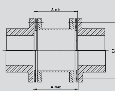
Axialverlagerung
