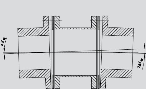
Winkelverlagerung
