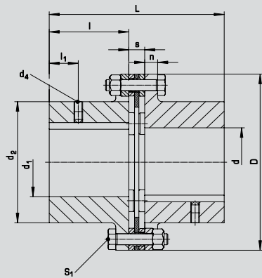
Bauform 1: einfach kardanisch
