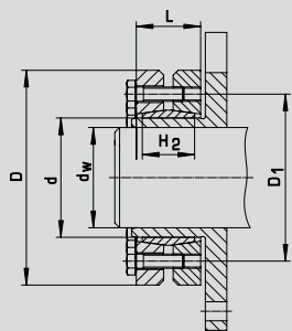
Schrumpfscheibe
