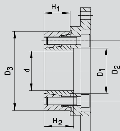
Bauform ...2: Spannsatz ArcOgrip Typ 356
