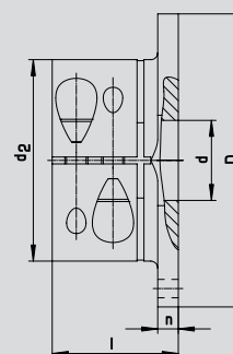
Klemmnabe
