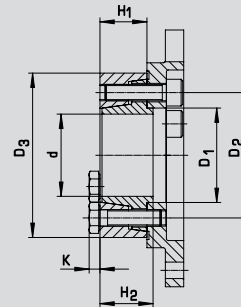
Spannsatz
