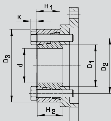
Bauform ...2: Spannsatz ArcOgrip Typ 354
