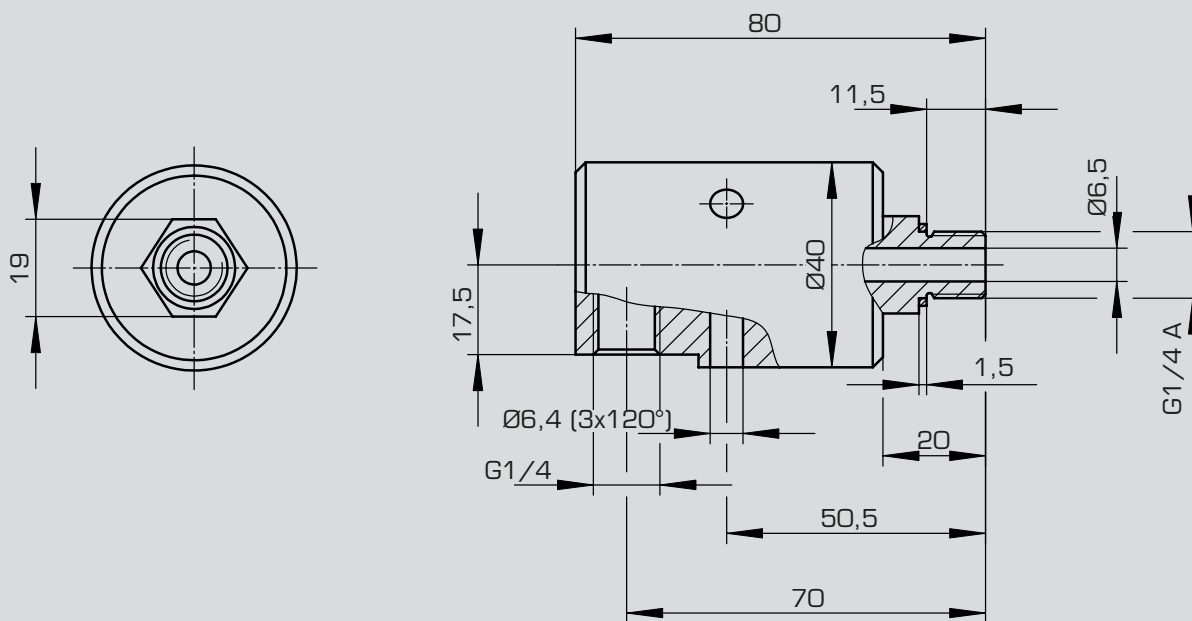
Dreheinführung Typ 598
