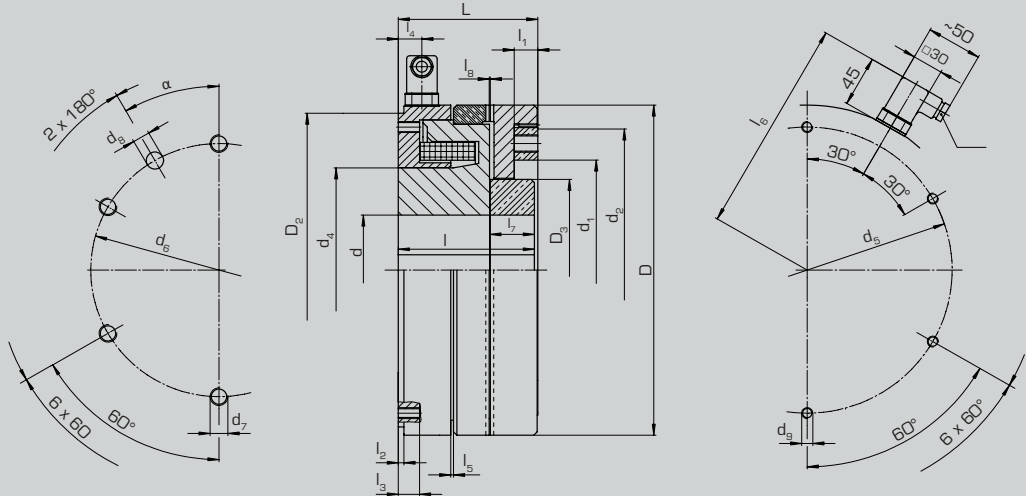
Zahnkupplung mit 2-poligem Steckanschluss
